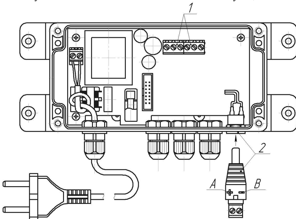
Рисунок В.1 – Расположение элементов коммутации УВ
