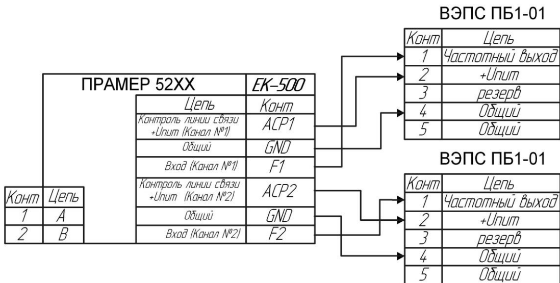
Рисунок В.4 – Схема подключения к ПР ВЭПС
