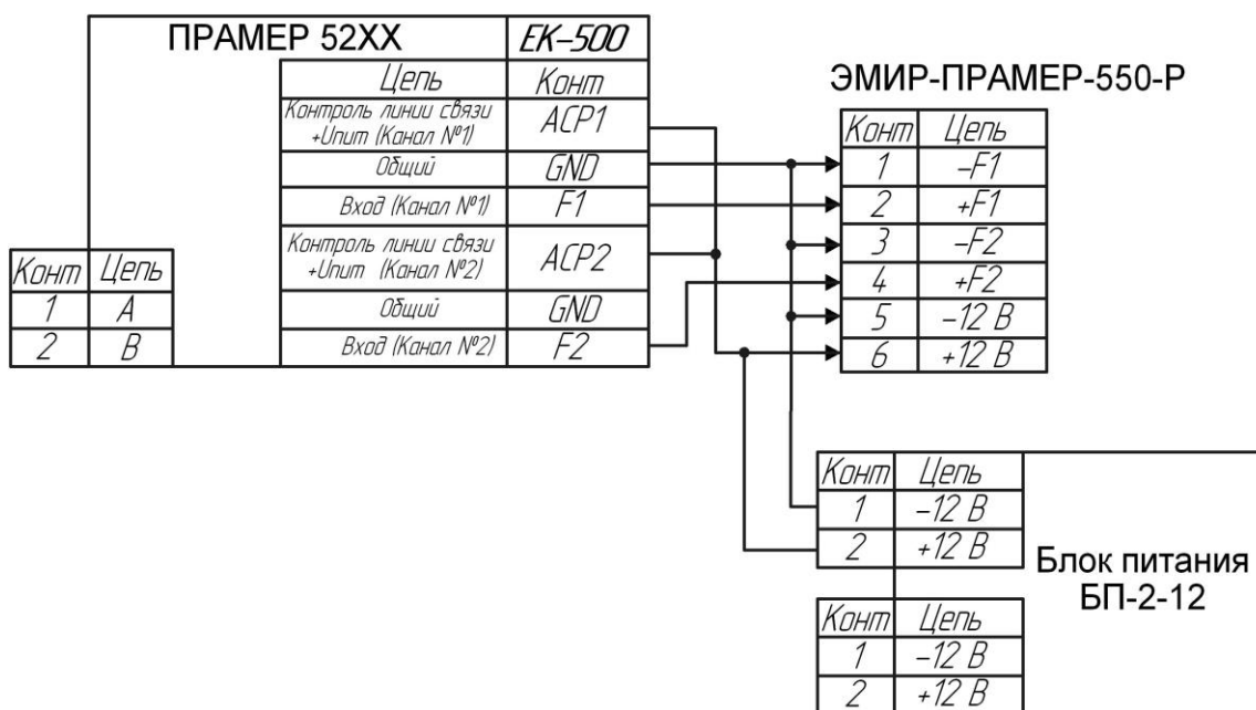
Рисунок В.6 – Схема подключения к ПР ЭМИР-ПРАМЕР-550 с реверсом
