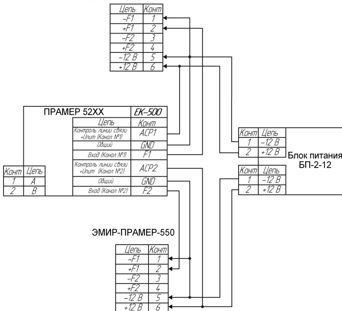
Рисунок В.5 – Схема подключения к ПР ЭМИР-ПРАМЕР-550
