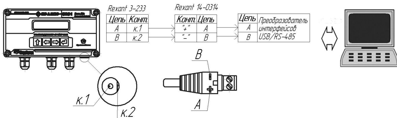
Рисунок Б.1 – Схема подключения к УВ в модификации с внешним разъёмом через цифровой интерфейс RS-485.
