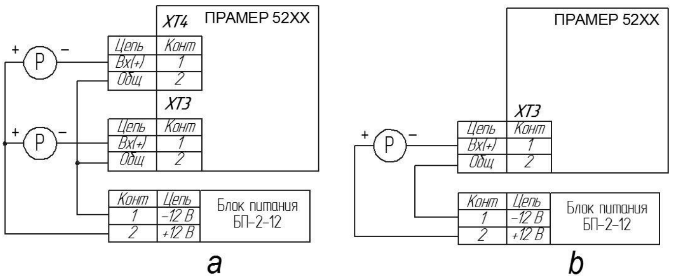
Рисунок В.7 – схемы подключения к УВ: a - двух ПД; b – одного ПД.
