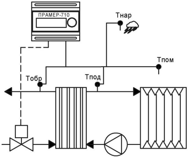
Управляемый теплообмен
