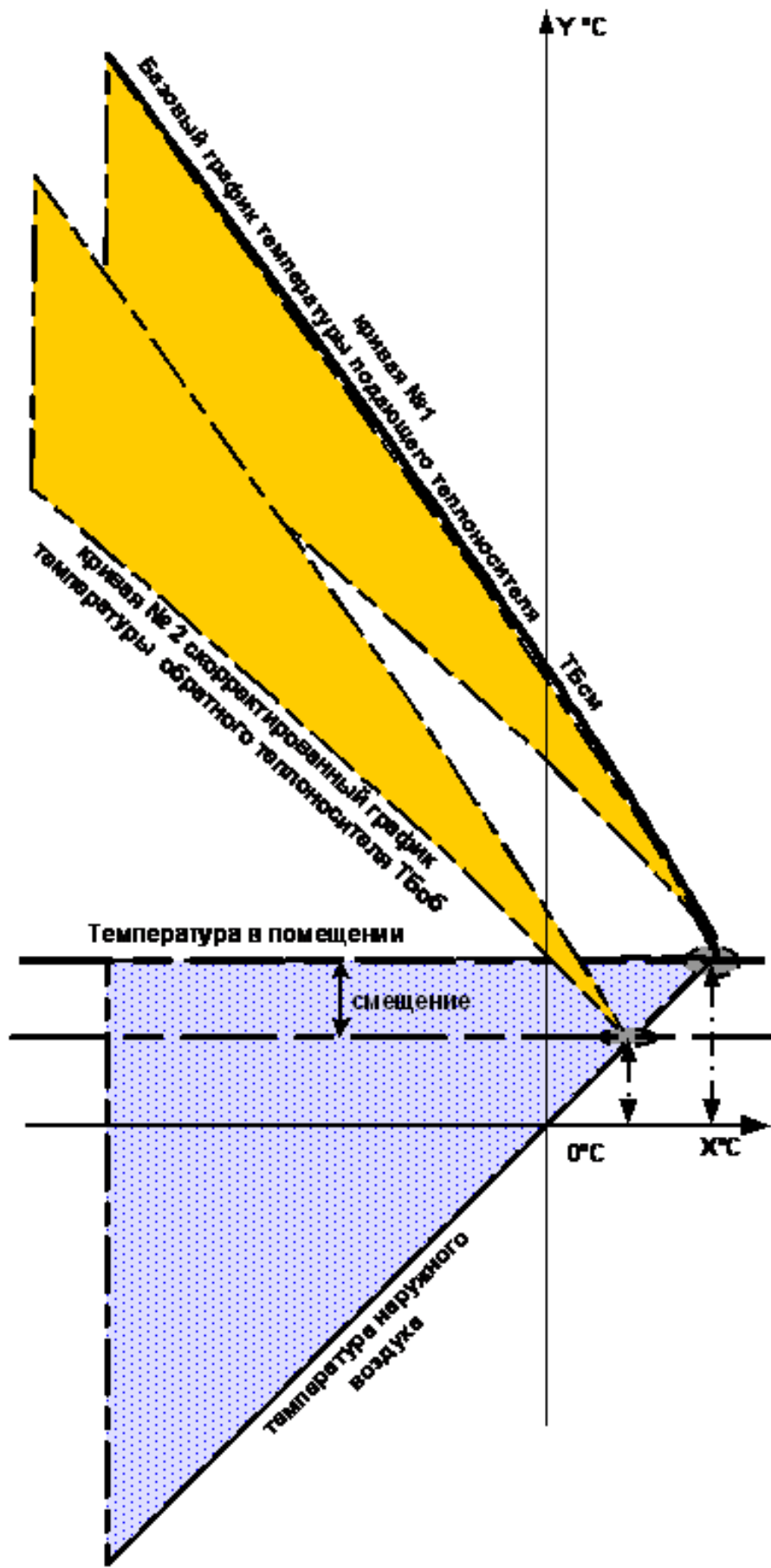
Рисунок 2. Температура комфорта
