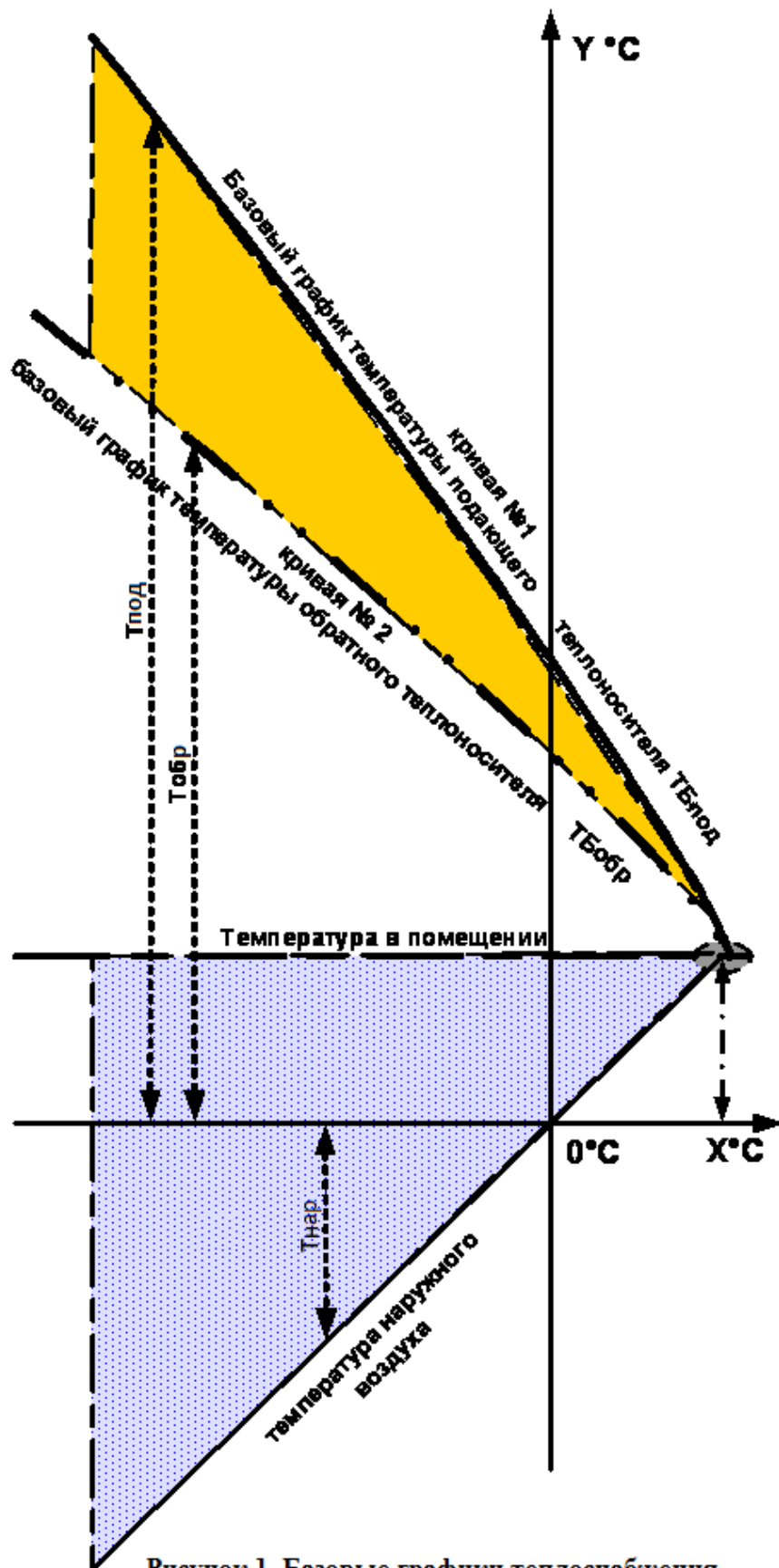
Рисунок 1. Базовые графики теплоснабжения
