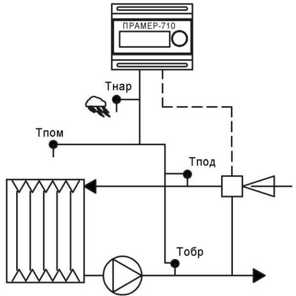
Электронный элеватор
