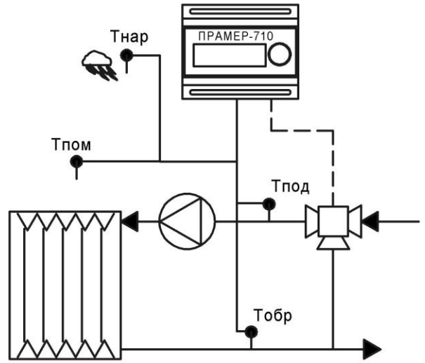
Схема смешения
