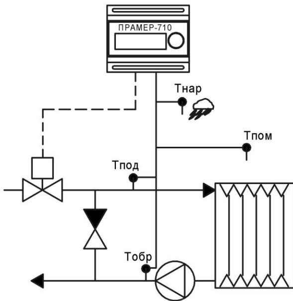
Схема смешения
