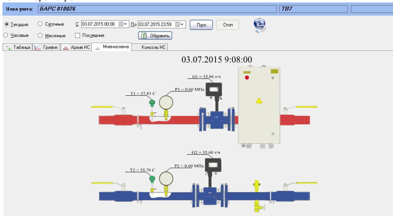
Рис. 9 Представление оперативных данных в виде мнемосхемы
