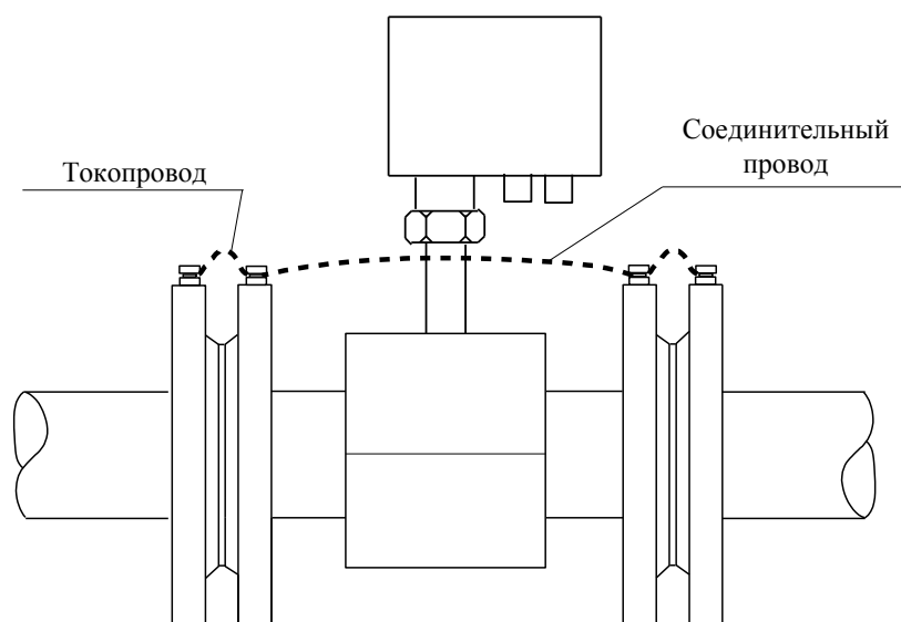
Рисунок 1 – Электрическое соединение фланцев преобразователя
