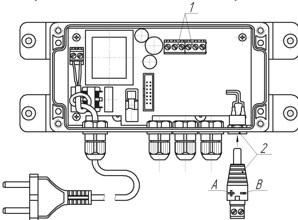
Рисунок В.1 – Расположение элементов коммутации УВ
