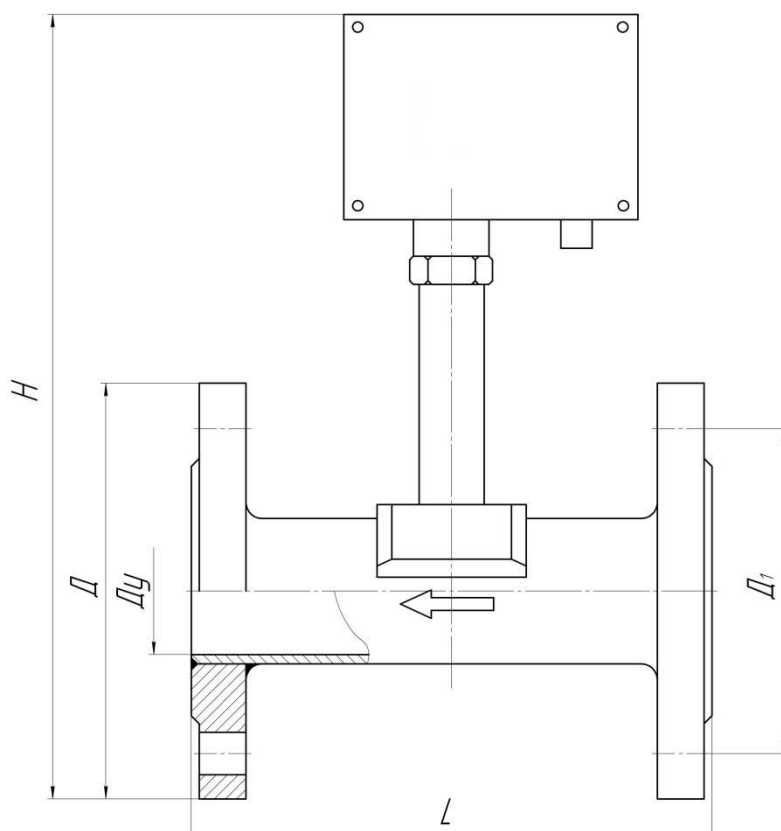
Рисунок Г.2 - Габаритные и присоединительные размеры ВЭПС-Р с
