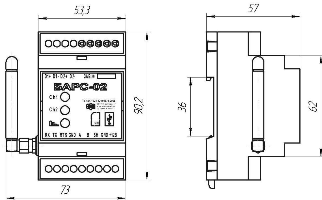
Рисунок А.1 – Габаритные и присоединительные размеры БАРС-02-Р-3-П
