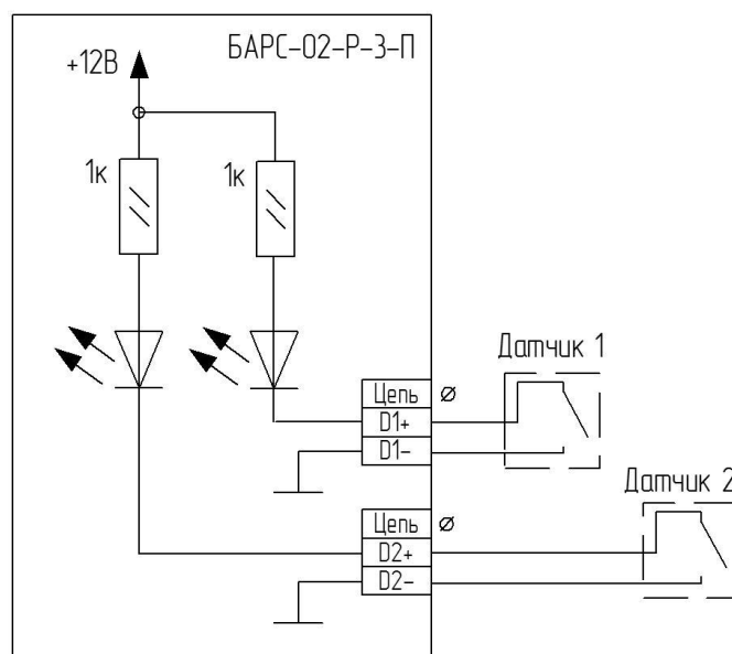
Рисунок Б.5 – Схема подключения дискретных датчиков
