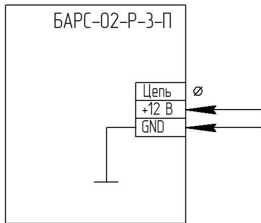
Рисунок Б.4 – Схема подключения источника питания
