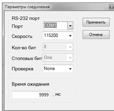
Рисунок 2 – Настройка параметров соединения
