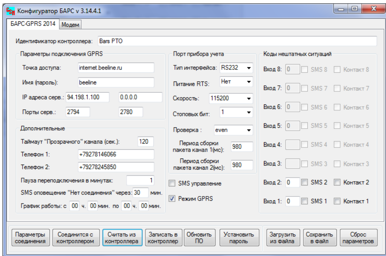
Рисунок 4 – Основное окно программы настройки для БАРС-02-Р-3-П
