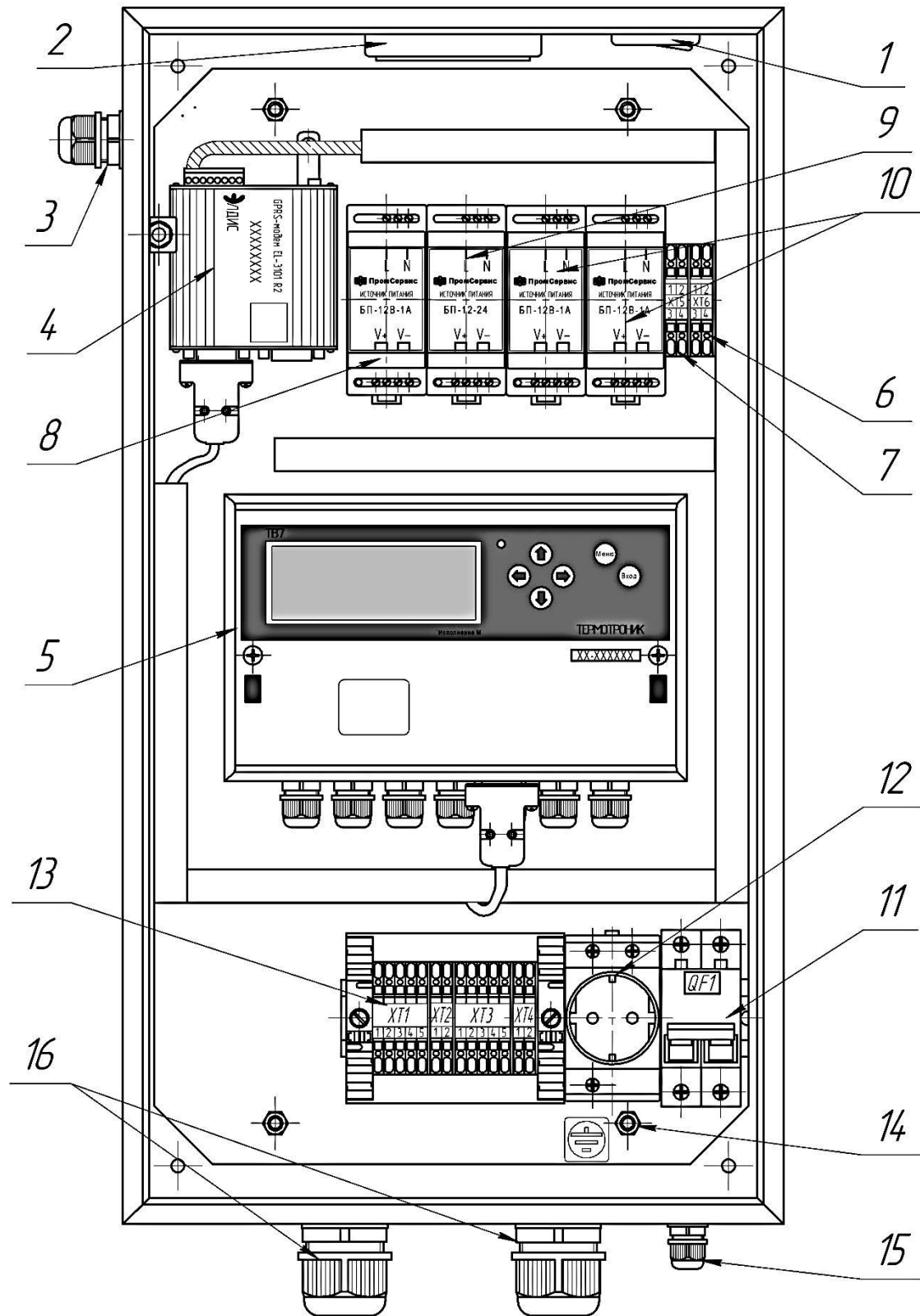
Рисунок 1 - Расположение составных элементов ШСУ-55-222-9:
