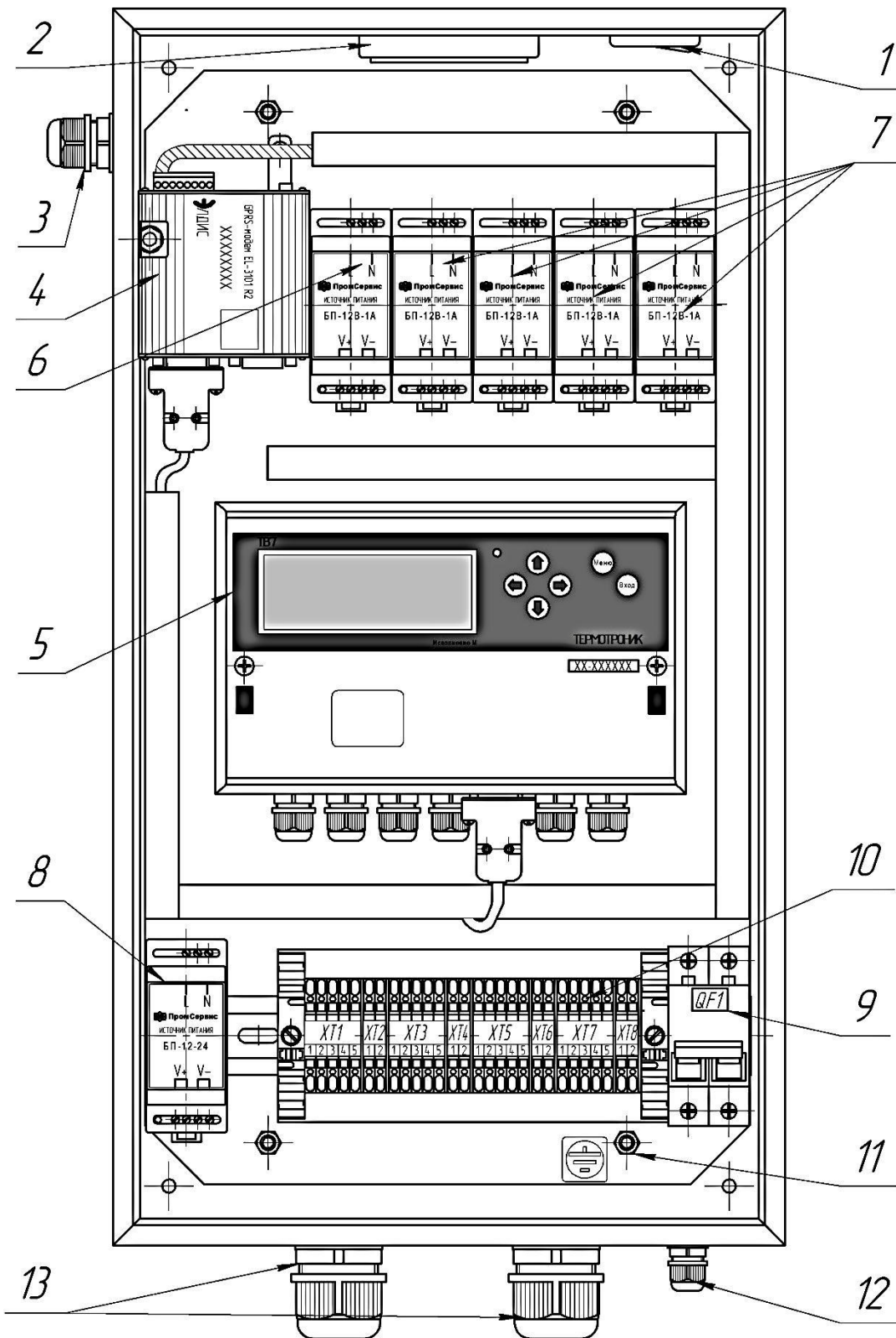
Рисунок 2 - Расположение компонентов внутри ШСУ-54-444-9:
