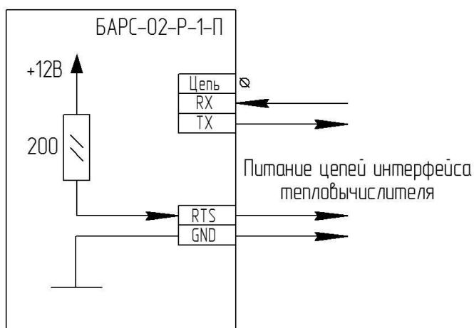
Рисунок Б.2 – Схема подключения к цепям интерфейса RS-232
